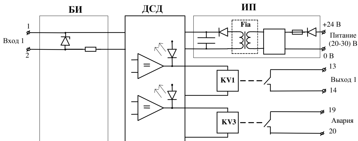
Рисунок 1 – Структурная схема преобразователя ET 121
