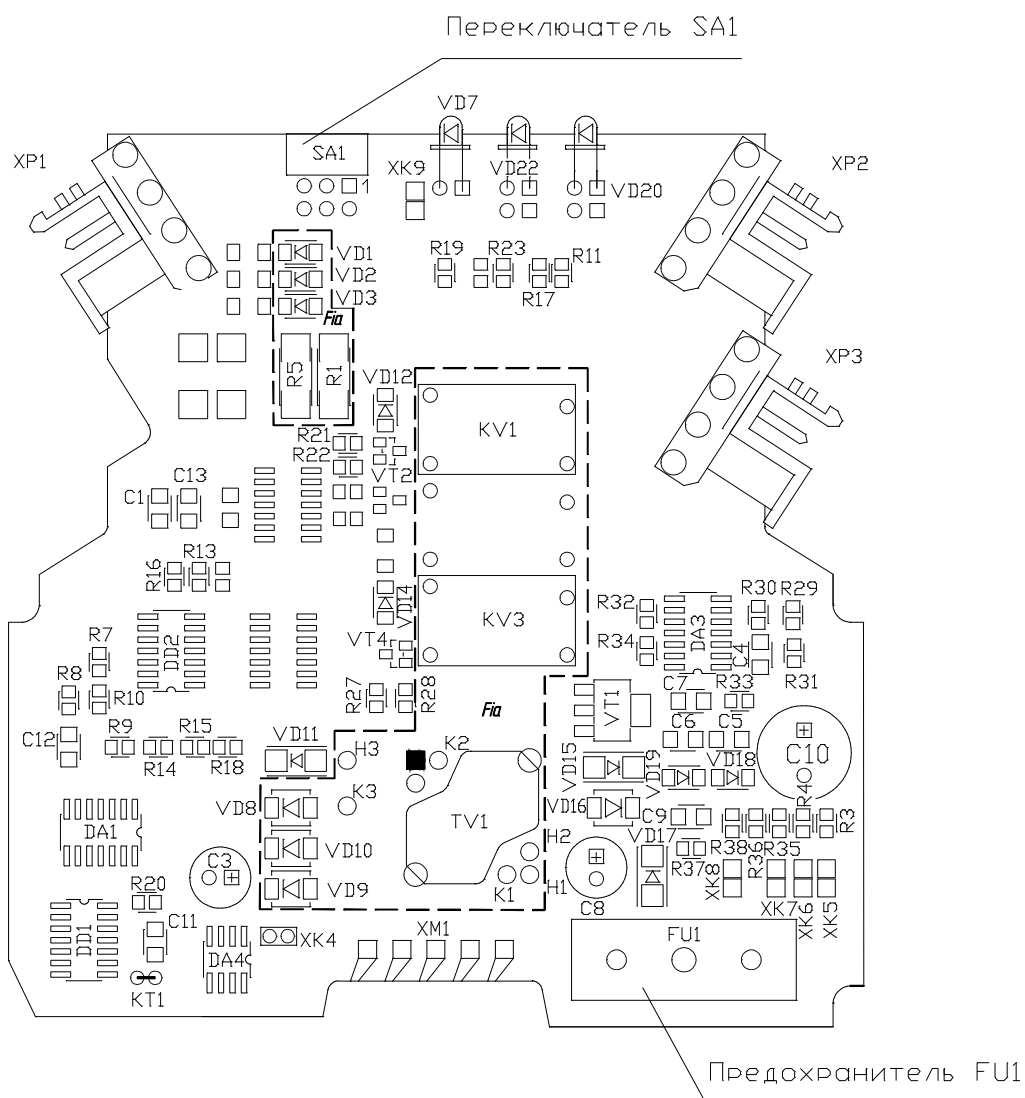
Рисунок Б.1 – Схема размещения элементов на плате преобразователя ET 121
