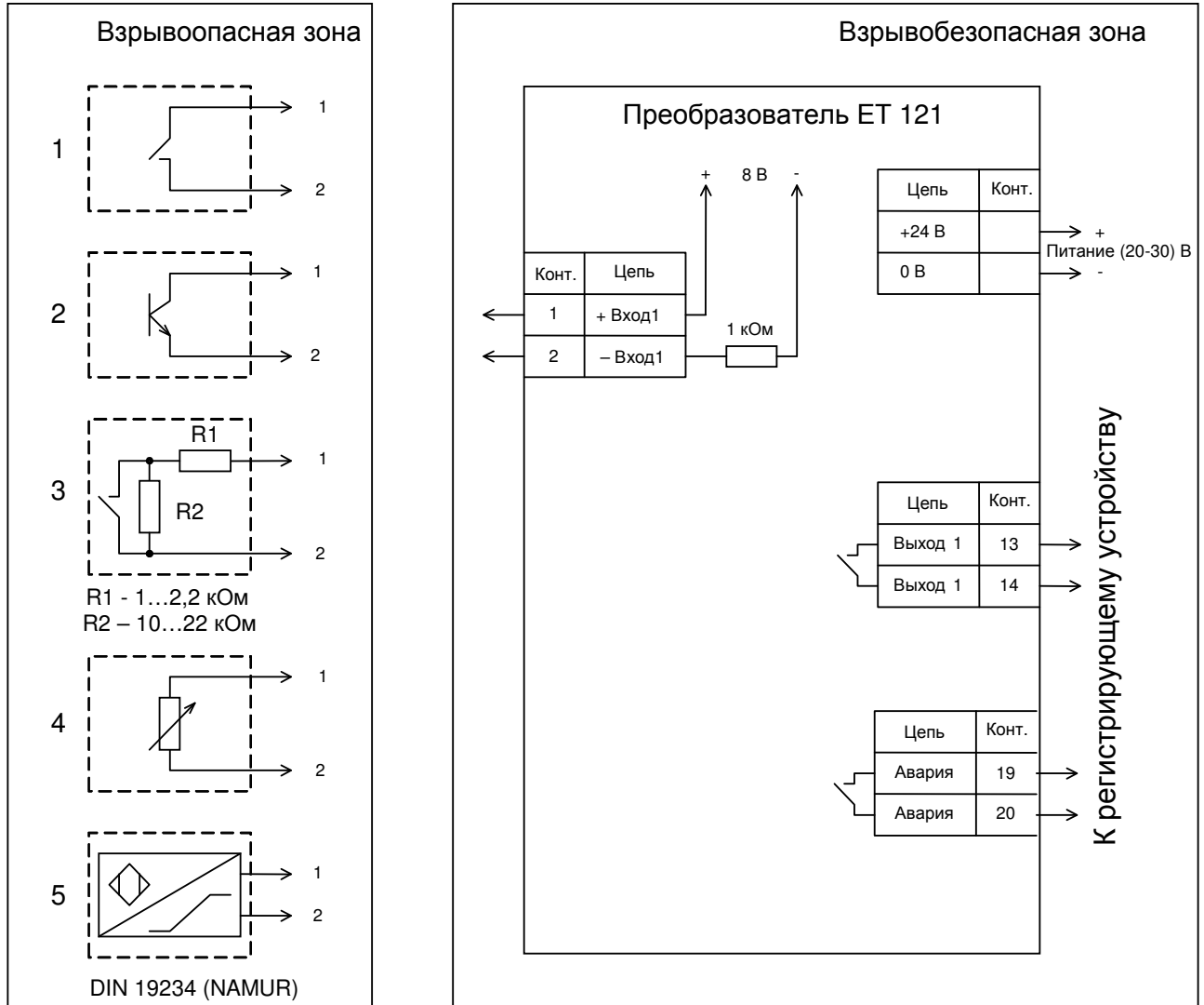
Рисунок В.1 – Схема подключения преобразователя ET 121
