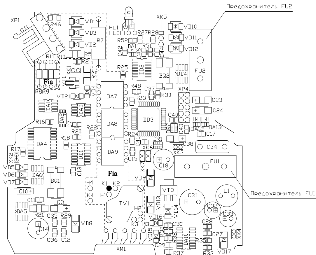
Рисунок Б.1 – Схема размещения элементов на плате преобразователя ET 481
