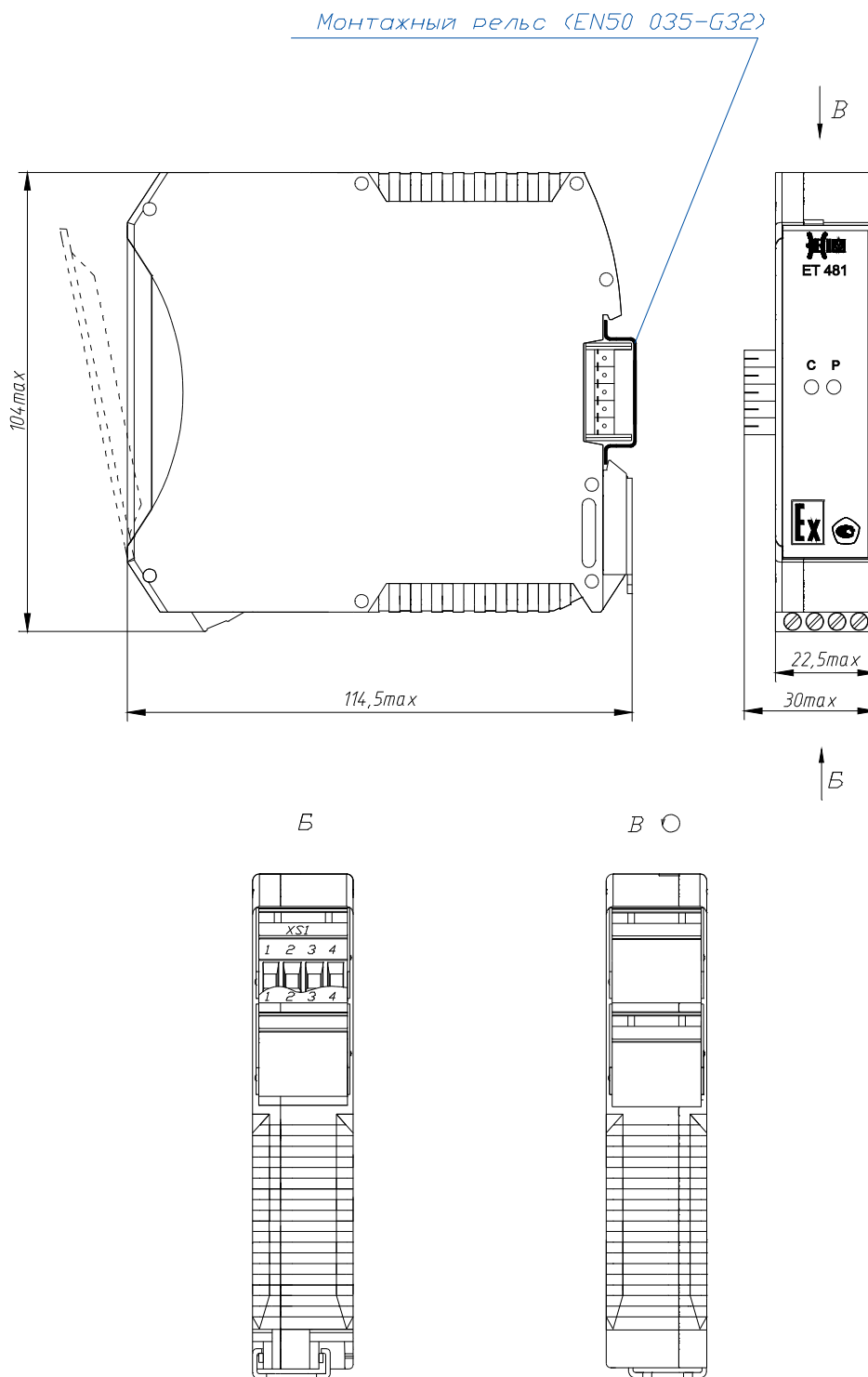
Рисунок А.1 – Габаритный чертеж преобразователя ET 481
