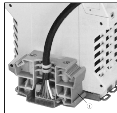
① Клипса E/ME TBUS NS35
