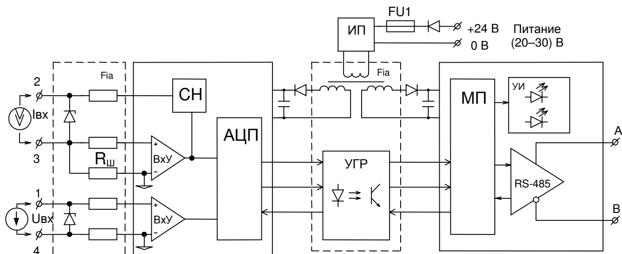
Рисунок 1 – Структурная схема преобразователя ЕТ 481
