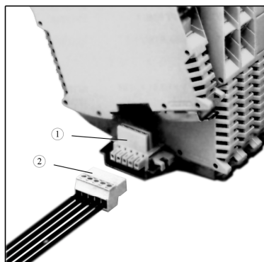
① ME 22,5 TBUS 1,5/5-ST-3,81 ② Вилка IМС 1,5 /5-ST-3,81AU Розетка МС 1,5/5-ST-3,81 AU
