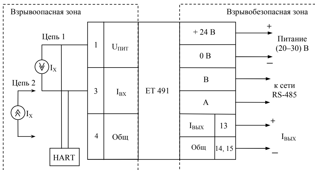
Рисунок В.1 – Схема подключения преобразователя ET 491
