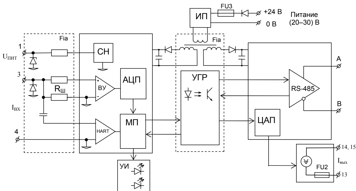
Рисунок 1 – Структурная схема преобразователя ET 491
