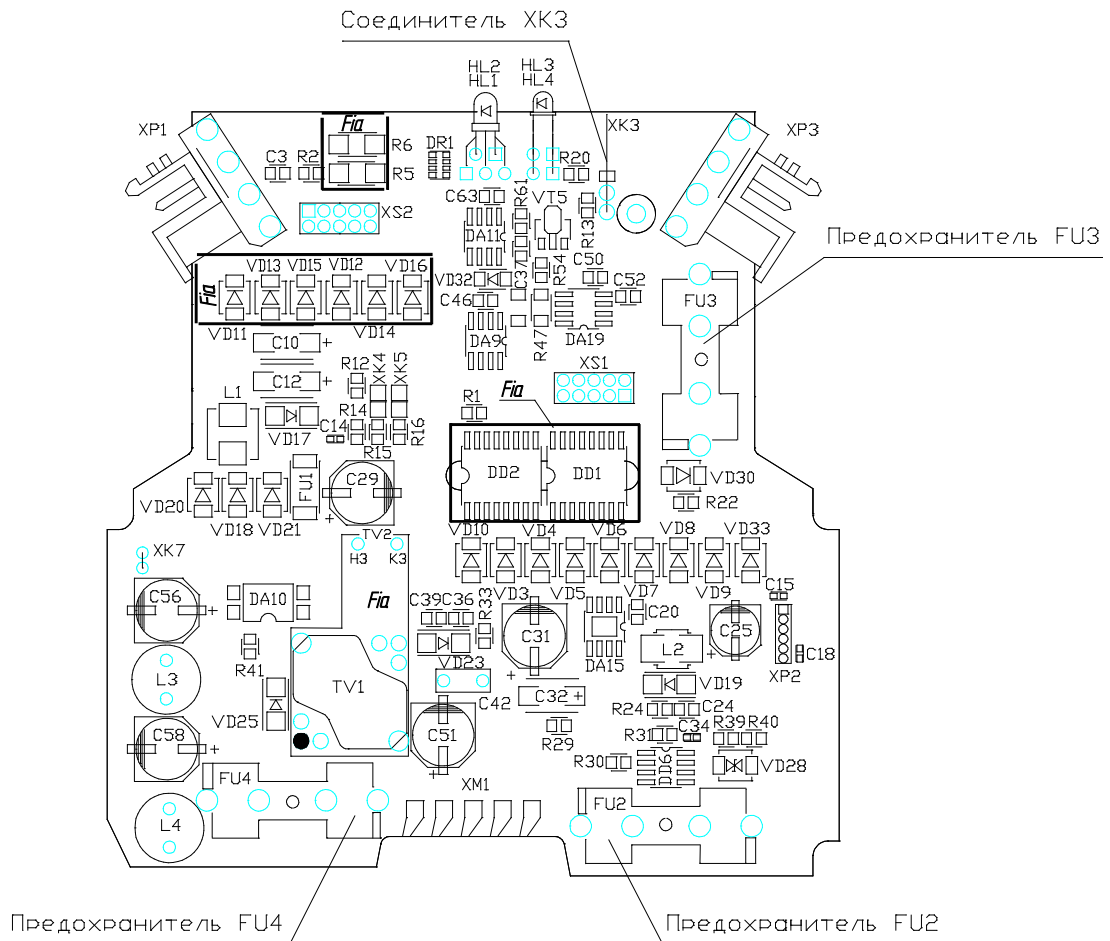
Рисунок Б.1 – Схема размещения элементов на плате МТ 7491А
