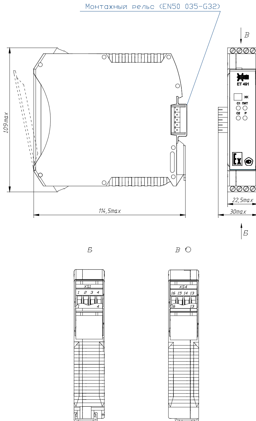
Рисунок А.1 – Габаритный чертеж преобразователя ET 491
