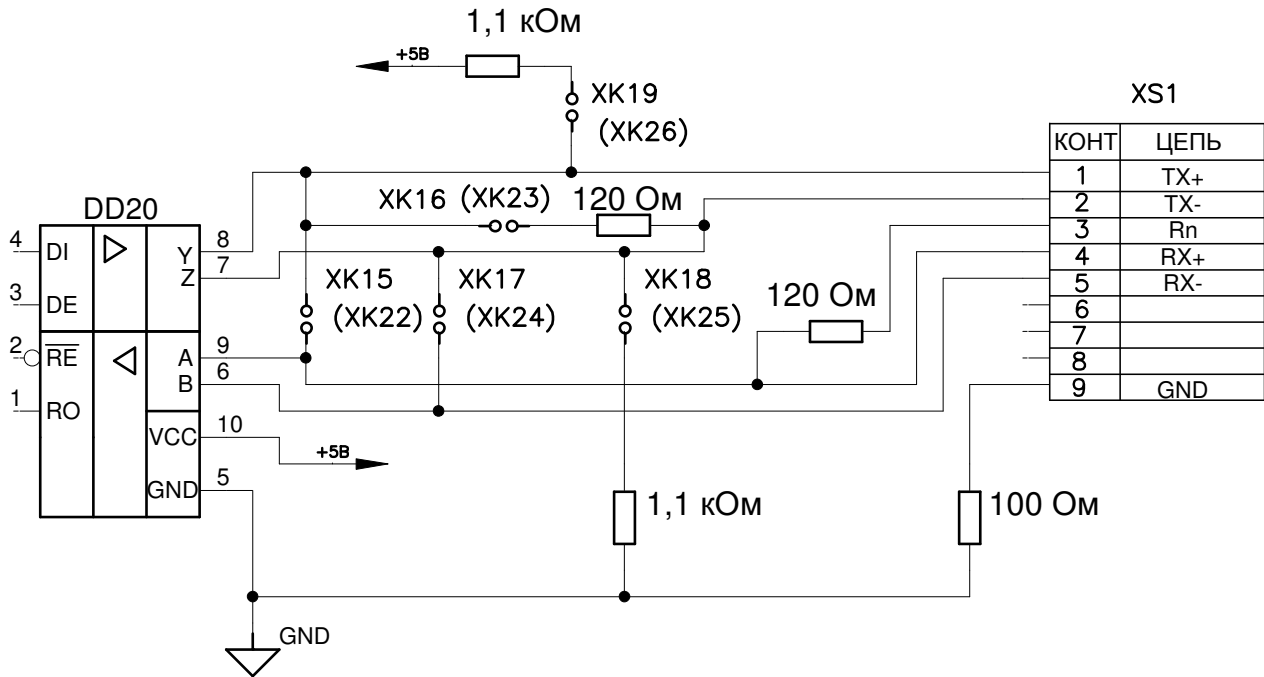
Рисунок В.1 – Схема выходных цепей интерфейса RS-485/RS-422
