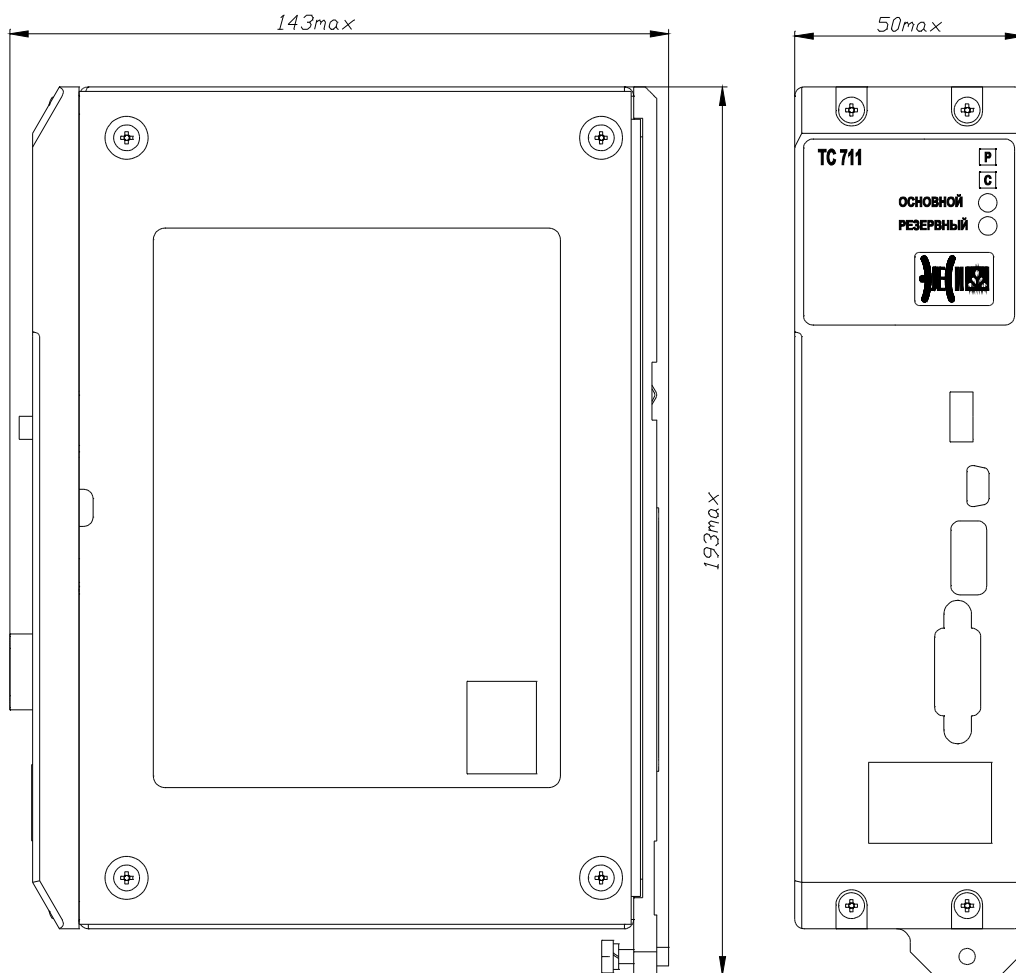
Рисунок А.1 – Модуль ТС 711. Габаритный чертеж
