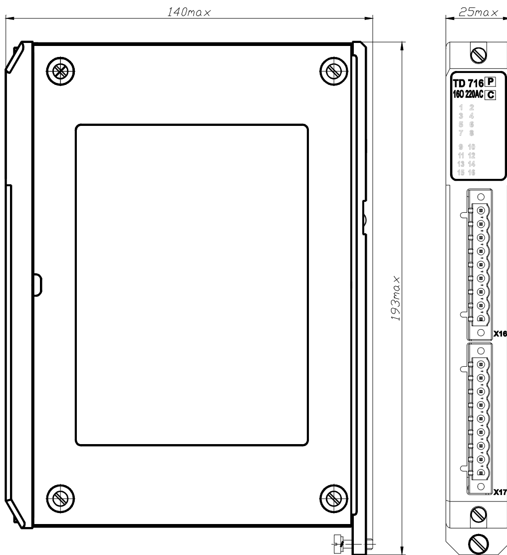
Рисунок А.1 – Внешний вид и габаритные размеры модуля TD 716
