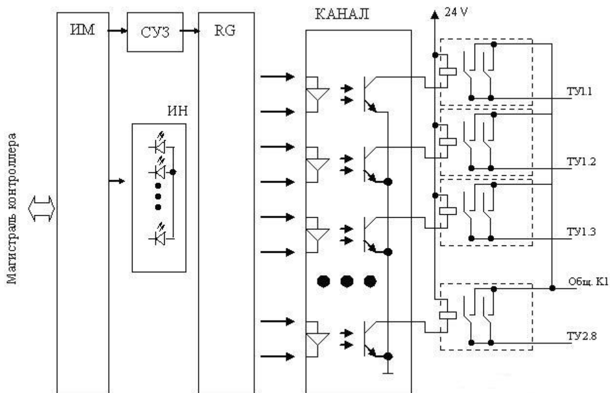
Рисунок Б.1 – Структурная схема модуля
