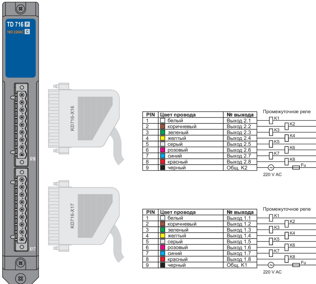
Рисунок 3 – Назначение контактов разъемов кабелей KD716-X16 и KD716-X17
