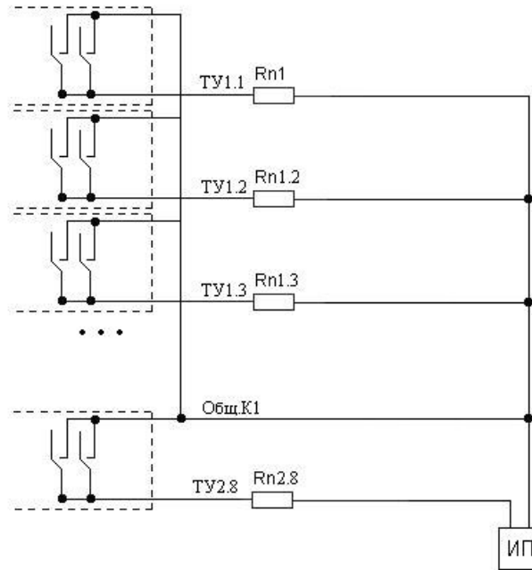
Рисунок 2 – Схема подключения модуля TD 716
